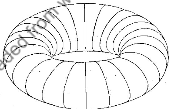
Fig. 27. Anchor-ring
