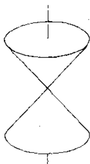
Fig. 28. Circular cone
