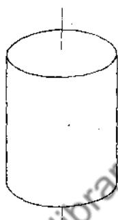
Fig. 29. Circular cylinder
